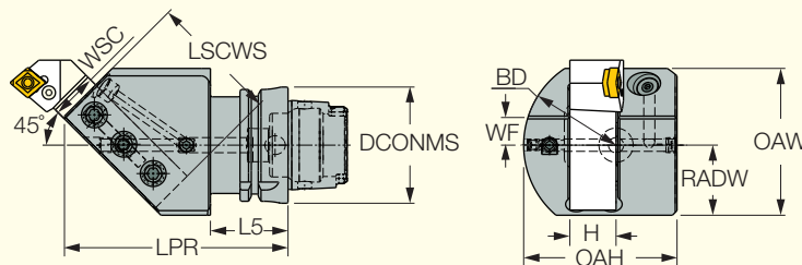
Abbildung zeigt rechtes Werkzeug in rechtem Adapter
